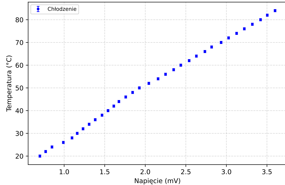
Termopara — Chłodzenie
